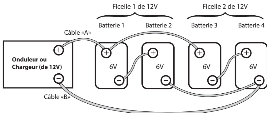
Figure 7.4 : Connexion série-parallèle
