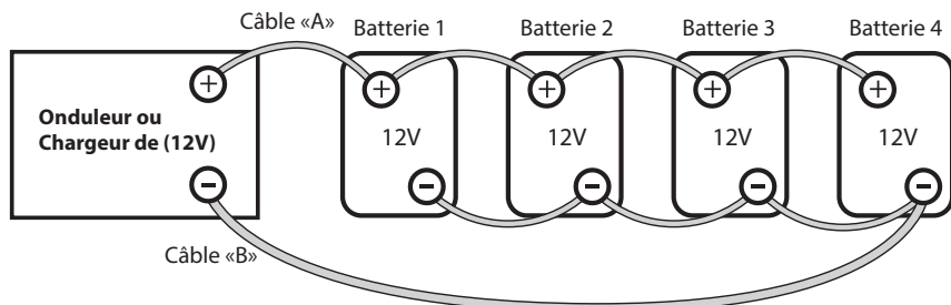
Figure 7.3: Connexion parallèle
